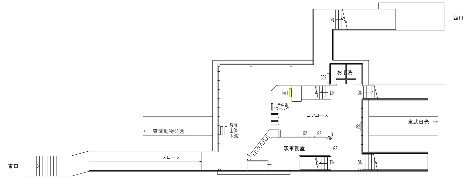
2Fコンコース平面図
