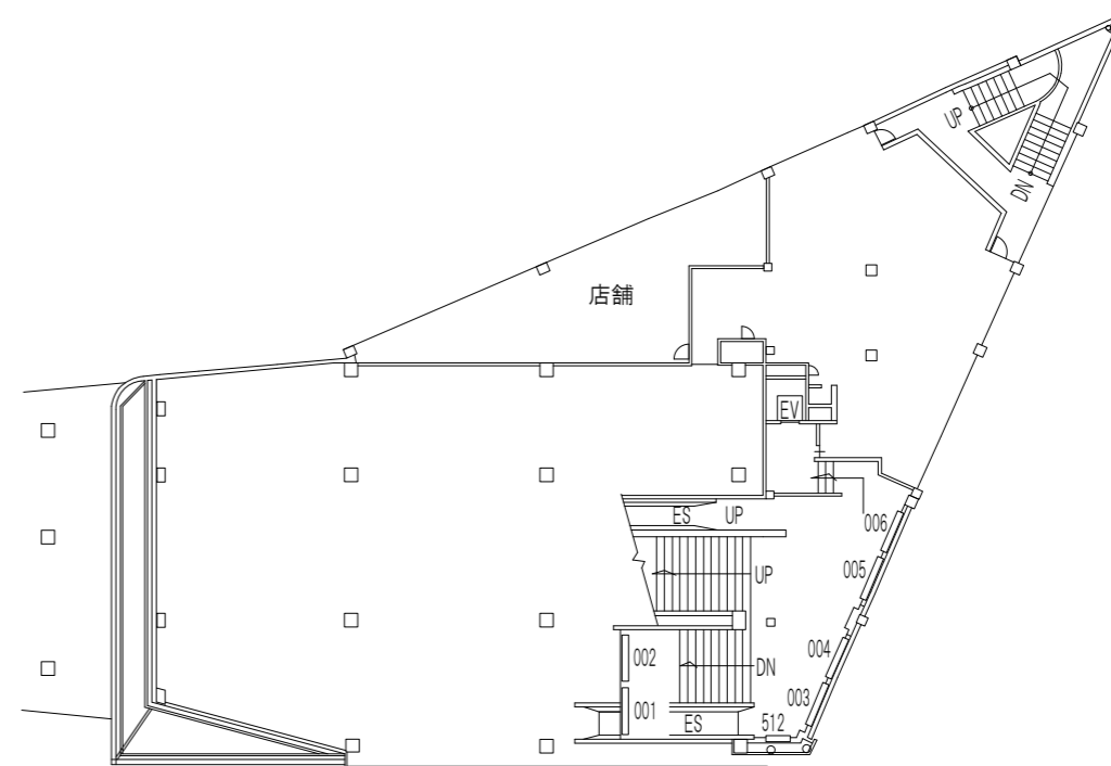
2階平面図
